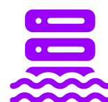
Data Lake
